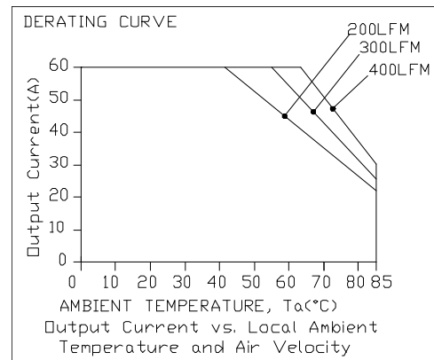
Vo=3.3V
