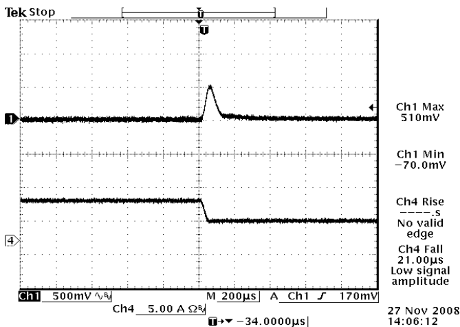
Vin=24V
