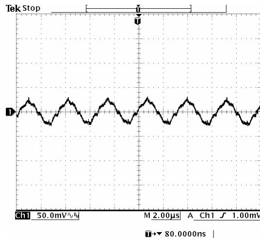
75 Vdc input
