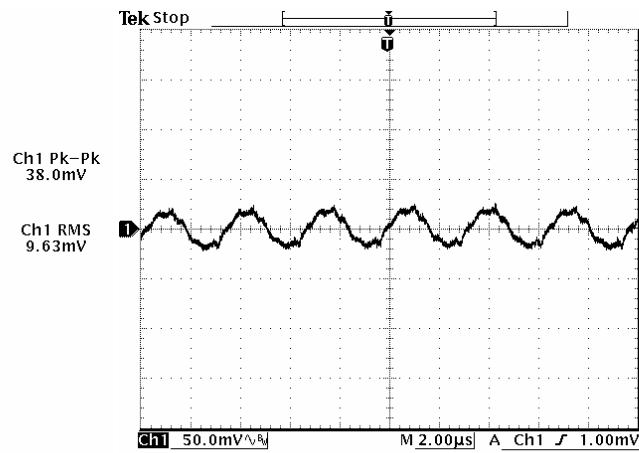
48 Vdc input
