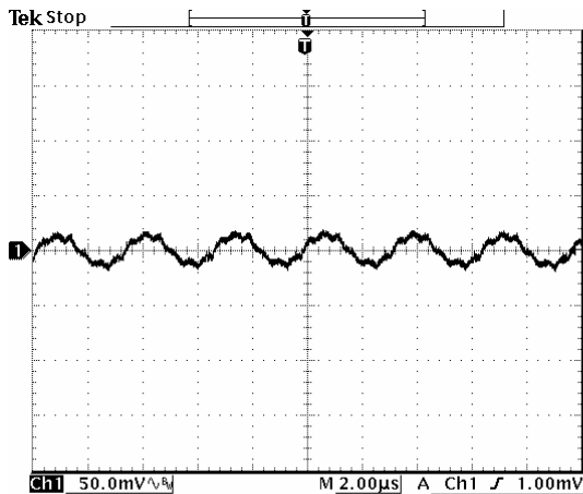
36 Vdc input
