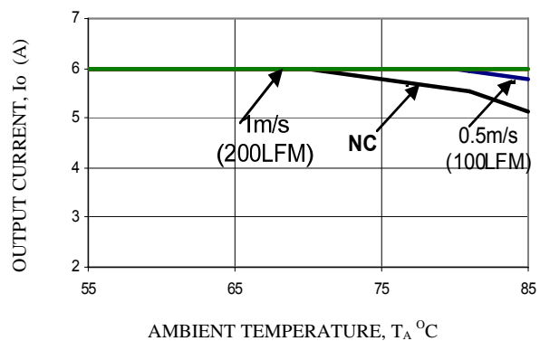
V_o = 5.0V
