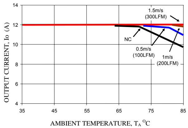
Vo=1.2V
