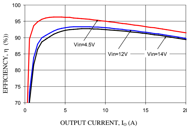
Vo=3.3V
