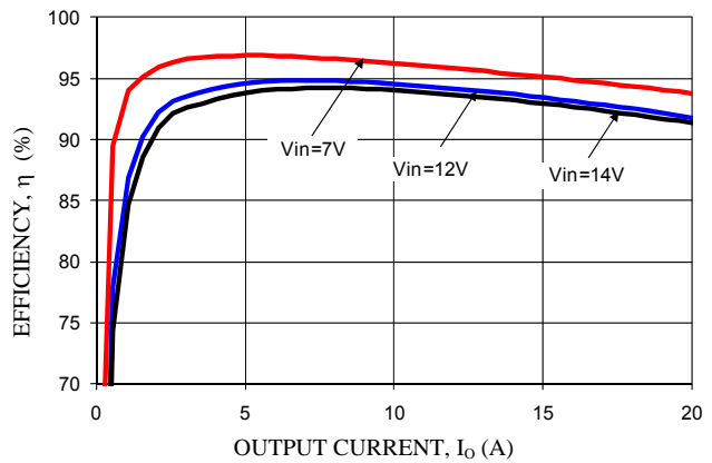
Vo=5.0V
