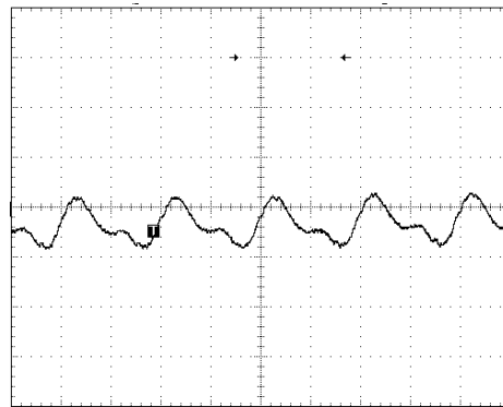
Vin=12V, Vo=1.2V, Io = Io,max
