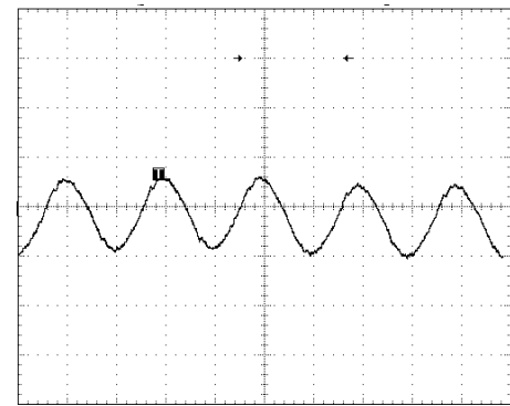
Vin=12V, Vo=2.5V, Io = Io,max
