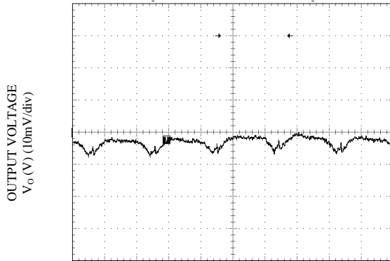
Vin=12V, Vo=0.69V, Io = Io,max
