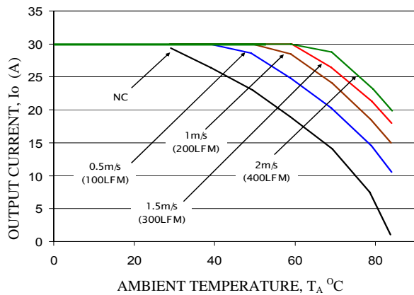
Vo=3.3V, Vin=12V
