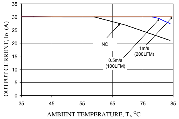
Vo=1.2V, Vin=12V
