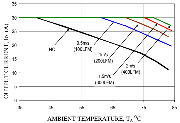
Vo=2.5V, Vin=12V
