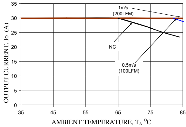
Vo=0.8V, Vin=12V
