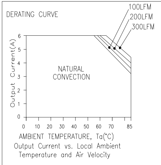
Vin=5 V, Vo = 3.3 V
