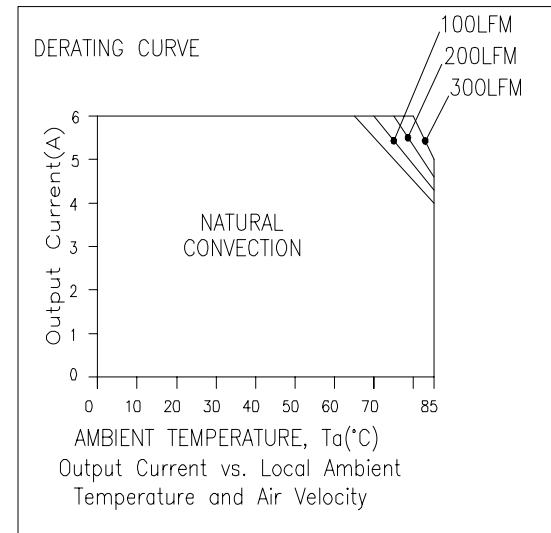
Vin=3.3 V, Vo = 0.75 V
