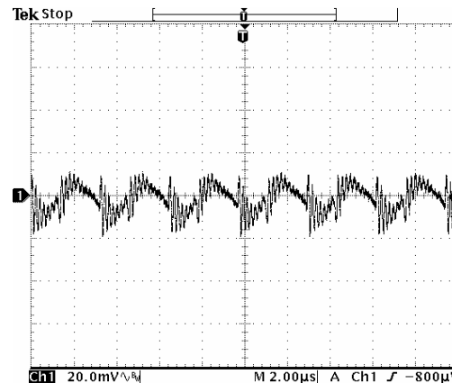
Vout=1.8 V
