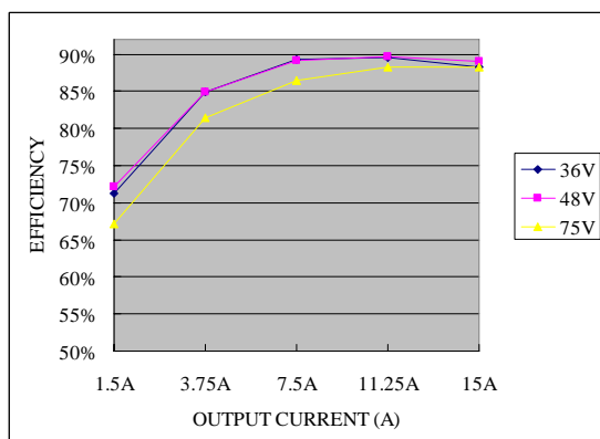
Vo=3.3 V
